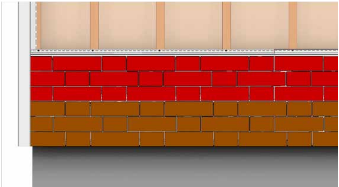
Рис. 17 Монтаж последующих рядов сайдинга
