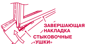
УСТАНОВКА ВЫРЕЗАННОЙ ЧАСТИ ПАНЕЛИ В ЗАВЕРШАЮЩУЮ НАКЛАДКУ
